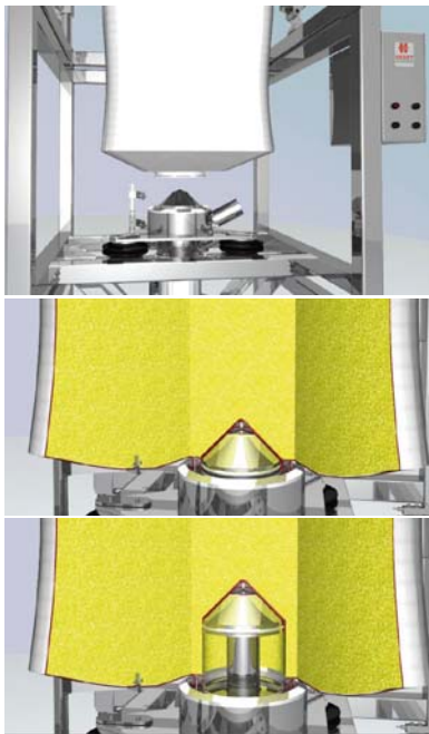
Automatisches Anschließen und Entleeren mithilfe der integrierten Austragshilfe (Heben und Senken des Verschlusskegels)
